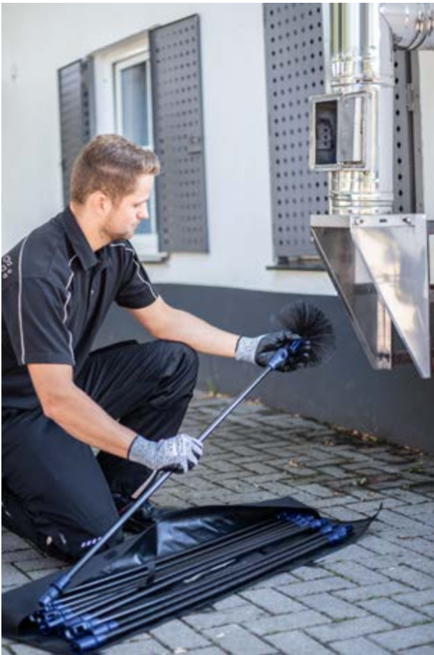
Mit nur einem Klick stecken Sie den Reinigungsvorsatz auf die Stange. Nicht benötigtes Werkzeug wird auf der geöffneten Tasche abgelegt, so dass der Arbeitsbereich sauber bleibt.
