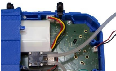
Abb. 16: Akku Wöhler A 450 angeschlossen, Sensoren sind entnommen, O 2 -Sensor Stecker und Gaswegschlauch sind noch angeschlossen.
