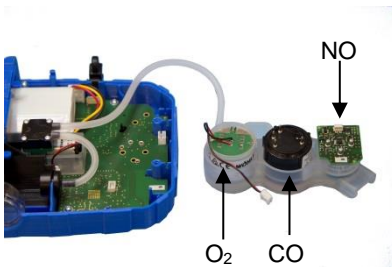
Abb. 12: Sensorhalten aus dem Gerät genommen
