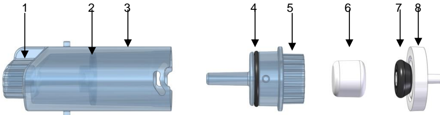
Abb. 4: Kondensatfalle
