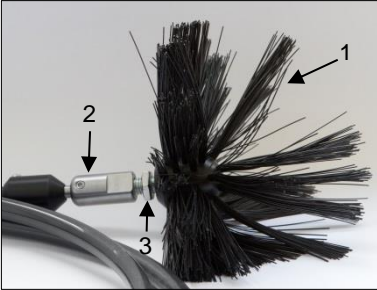
Abb. 2: Reinigungsaufsatz (1), Aufnahme mit M10 Innengewinde (2) und Kontermutter (3)
