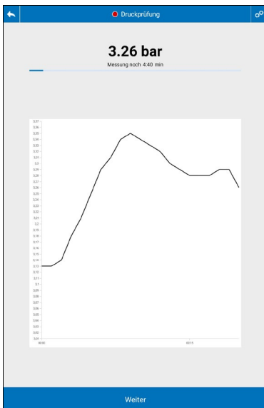
Abb. 17: Anzeige des Druckverlaufs während der Messung
