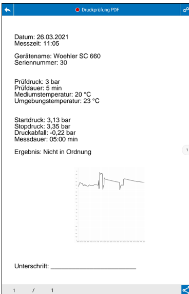
Abb. 19: PDF-Protokoll
