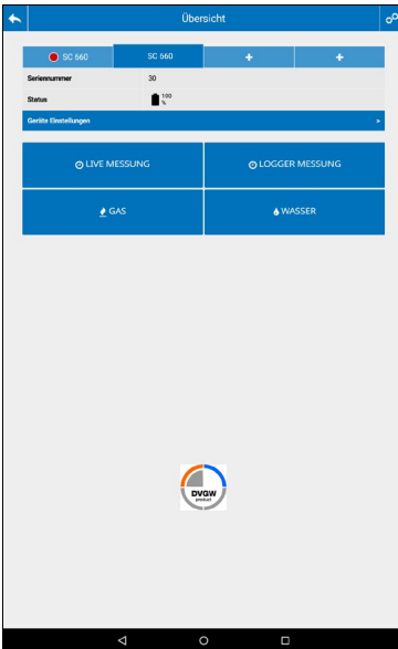
Abb. 4: Übersichtseite
