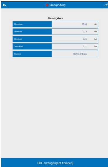
Abb. 18: Ergebnisanzeige Druckprüfung mit Wasser
