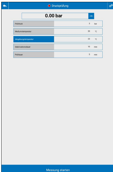
Abb. 16: Voreinstellungen Druckprüfung an Wasserleitungen mit Wasser
