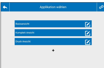
Abb. 9: Live-Ansichten (Beispiel)
