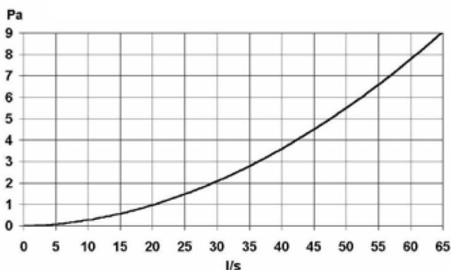
Abb. 6: Druckverlust über das SWF 236
