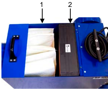
Image 11: Compartiment des filtres avec prefiltre (1) et microfiltre(2)
