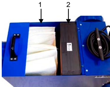
Abb. 11: Filterfach mit Vorfilter (1) und Feinfilter (2)
