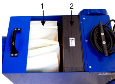
Afb. 35: Filtervak met voorfilter (1) en fijnfilter (2)
