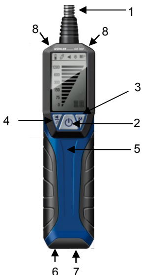
Afb. 23: Gasvoeler
